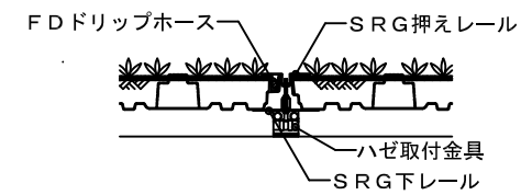
C部詳細図
